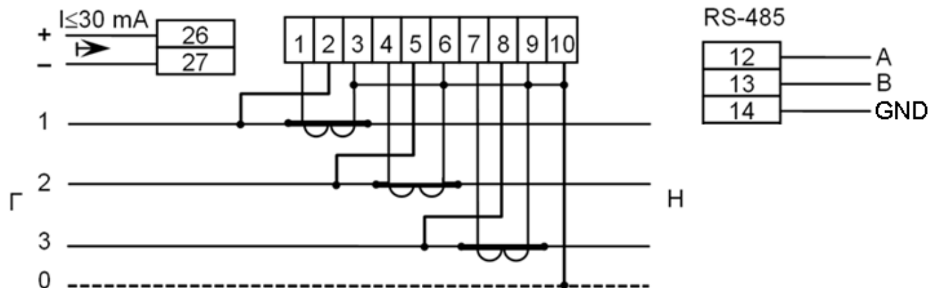
Схема включения счетчиков СЕ307 R33.043.ОА
