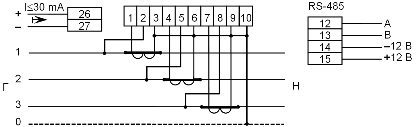
Схема включения счетчиков СЕ307 R33.043.О, СЕ307 R33.043.ОА.N
