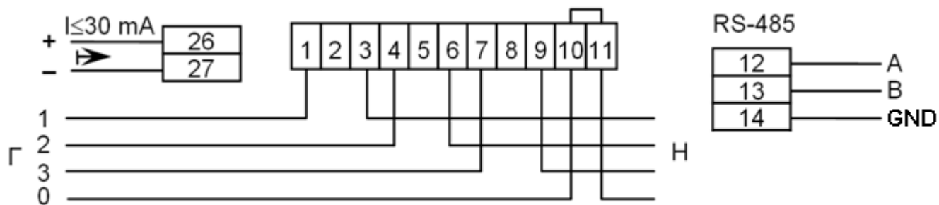
Схема включения счетчиков СЕ307 R33.145.0А, СЕ307 R33.146.0А
