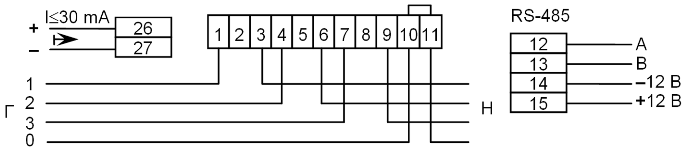
Схема включения счетчиков СЕ307 R33.043.ОА
