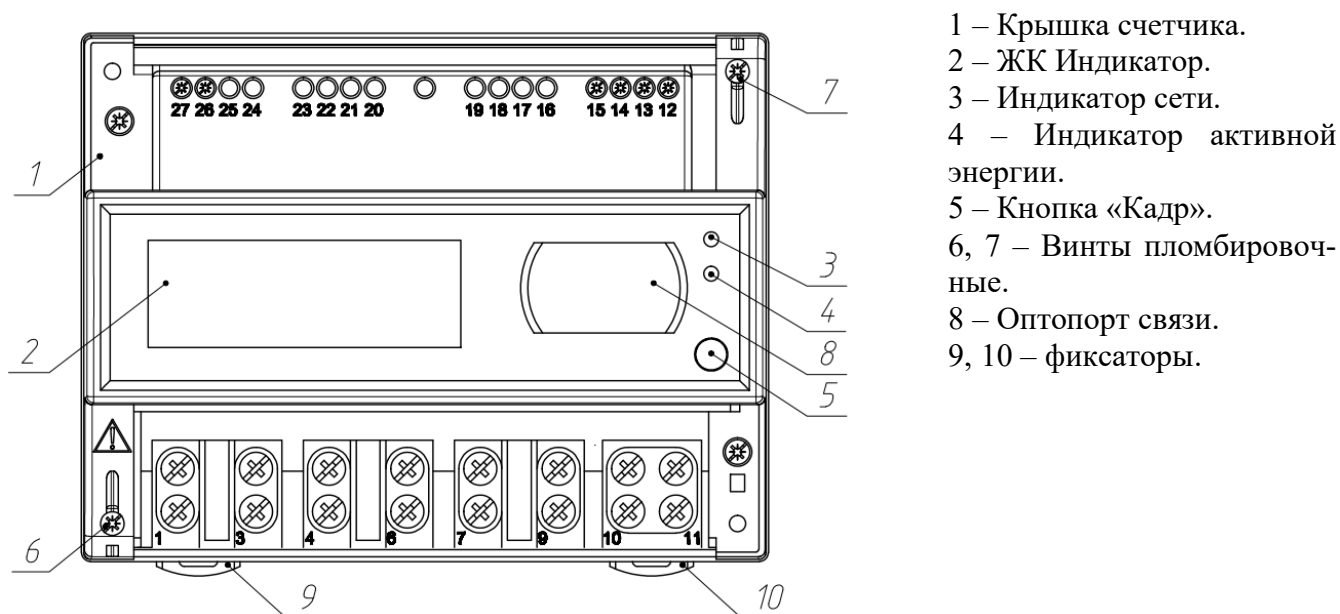
Рисунок 2 – Общий вид счетчика
